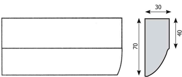
Listwa wykończeniowa profil A
