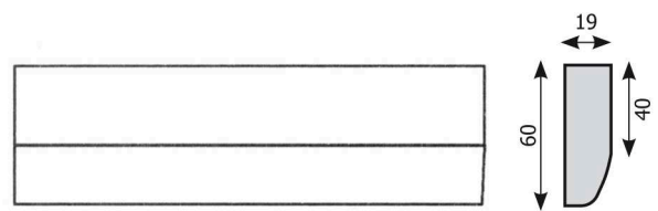
Listwa podszafkowa profil A
