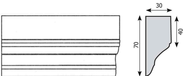
Listwa wykończeniowa profil B
