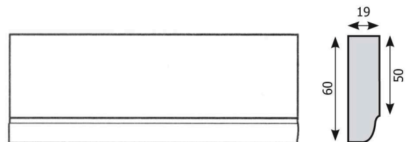
Listwa podszafkowa profil B
